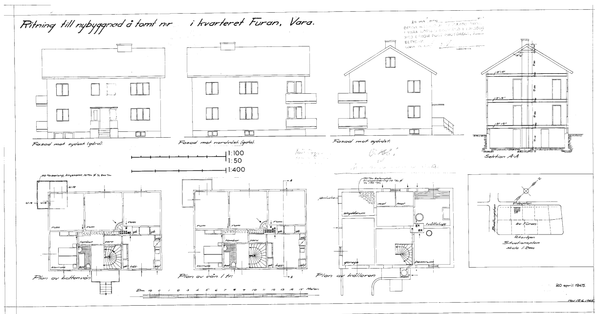
Kvarteret Furan nybyggnadsritning 1945, exempel på en tvåfamiljs villa som uppfördes i Vara runt 1940-talets mitt. Majoriteten av byggnaderna av samma karaktär inom tätorten är idag mycket förändrade. Ritning: Vara Kommun.
