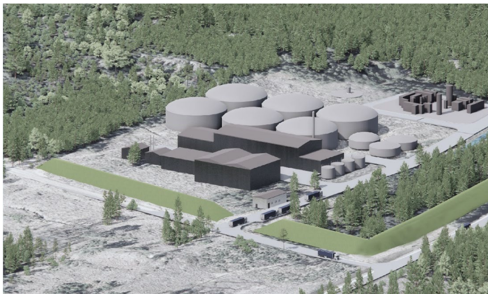
Bilden ovan är en översiktsbild som redovisar en möjlig utbyggnad av biogasanläggning med blick mot nordväst. Bild: Tengbomgruppen AB.
