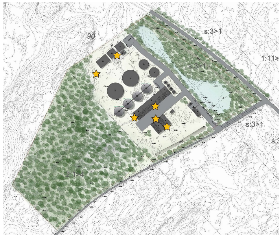
Illustrationen ovan redovisar av möjlig placering av olika anläggningsdelar inom verksamhetsområdet. Stjärnmarkeringarna redovisar utsläppspunkter. I detaljprojektering kan ändringar komma att ske. Bild: Rönnöls Miljökonsult.
